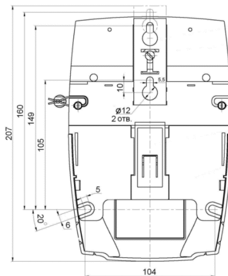
Рисунок 2.2 – Установочные размеры коммуникатора
