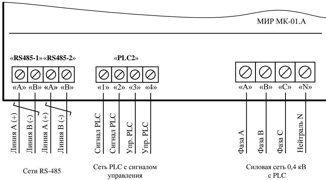
Рисунок 7.2 – Схема подключения внешних цепей коммуникатора с питанием от силовой сети переменного тока напряжением 0,4 кВ (модификации с символами «Р», «P1», «P2», «P3», «2R» в коде коммуникатора)
