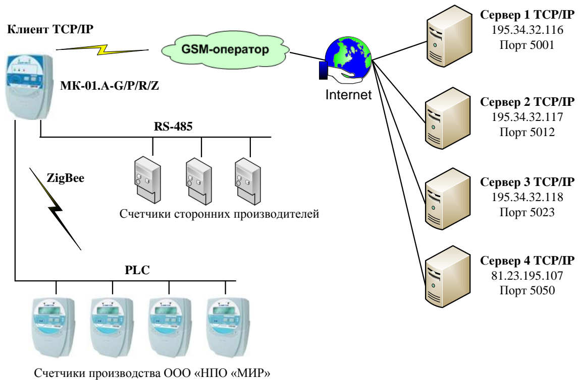
Рисунок 8.45 – Пример использования коммуникатора в качестве клиента TCP/IP
