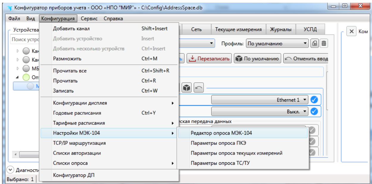
Рисунок 8.26 – Вход в редактор опроса МЭК-104
