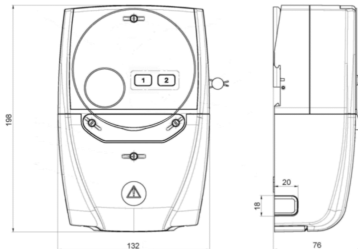
Рисунок 2.1 – Габаритные размеры коммуникатора
