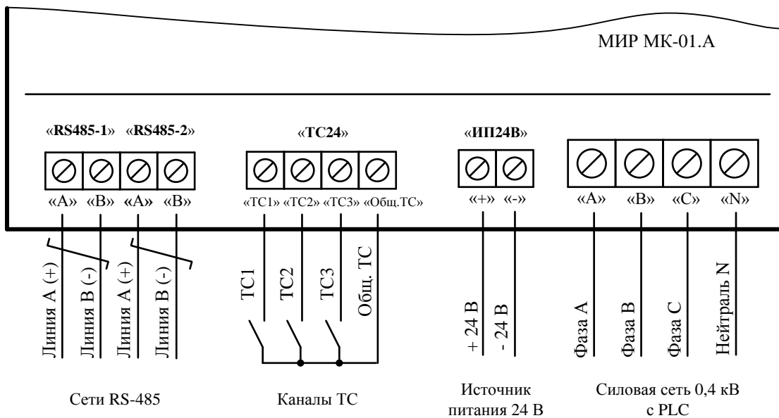
Рисунок 7.3 – Схема подключения внешних цепей коммуникатора с питанием от источника постоянного тока напряжением 24 В (модификации с символами «Р», «P2», «2R», «3TC24» в коде коммуникатора)
