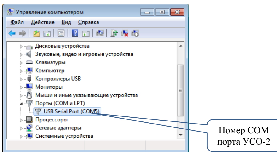
Рисунок 8.3 – Номер COM-порта УСО-2
